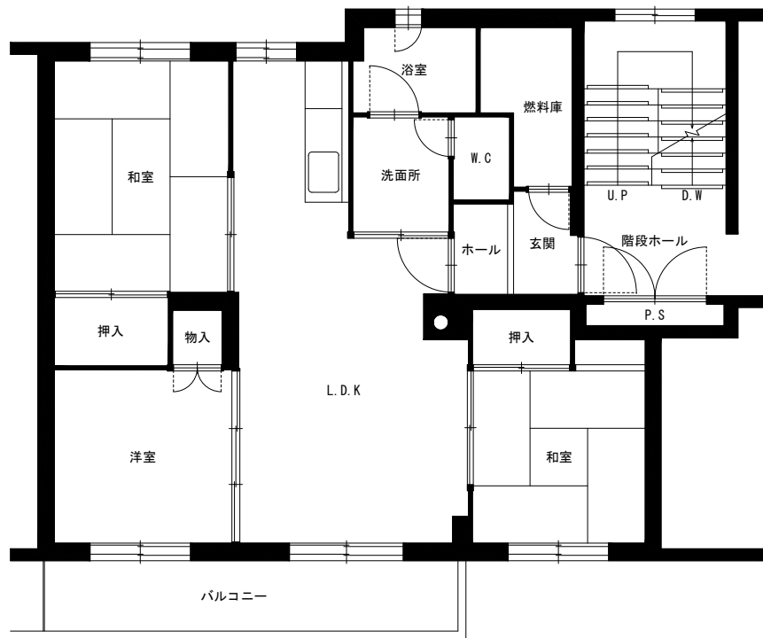
メロディー R-1 3LDK R-TYPE
